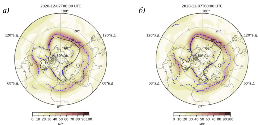
Рисунок 7 – Широтно-долготное положение ядер СТ (синие пунктирные линии) и положение ПВФЗ (черные линии) по значению характерной изогипсы данных реанализа NCEP/NCAR (а) и JRA-55 (б) в срок 00 UTC 7 декабря 2020 г. Заливкой представлена средняя скорость ветра слоя 500–100 гПа.
