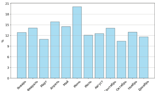
Рисунок 6 – Значения параметра P_i для периода 1980–2023 гг. по данным реанализа JRA-55.
