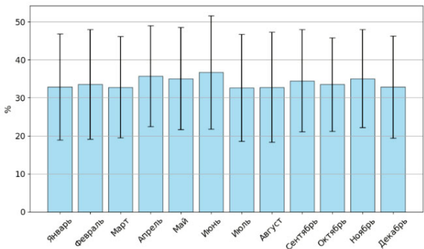
Рисунок 5 – Среднемесячные значения P_{EV} , ST_{A-E} и SKO для периода 1980–2023 гг. по данным реанализа JRA-55.
