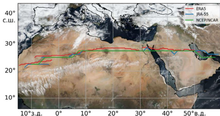
Рисунок 2 – Широтно-долготное положение ядер ССТ в полях ветра реанализов ERA5, JRA-55 и NCEP/NCAR в срок 12 UTC 22 января 2019 года.
