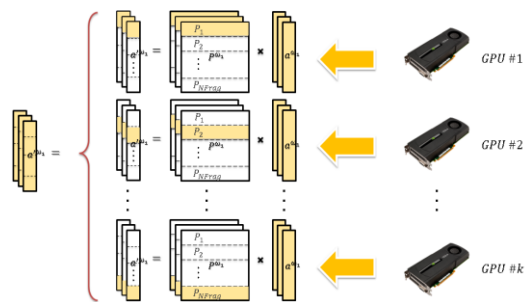
Рисунок 4. Схема реализации компоненты МатрицаРаспространения для GPUs.
