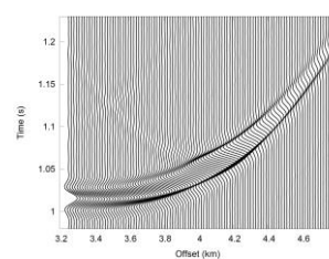
Рисунок 12. Двукратное преломление в приёмниках на «линия 1».
