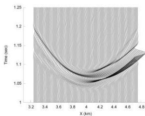
Рисунок 11. Поле источника в приёмниках на «линия 1».
