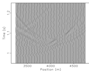
Рисунок 20. Разница сейсмограмм МНКВ и МКР.
