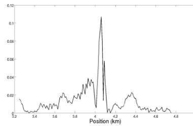
Рисунок 22. Относительное отклонение КДО МНКВ от КДО МКР.
