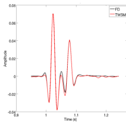
Рисунок 18. Наложение трасс МНКВ (красная) и МКР (чёрная).
