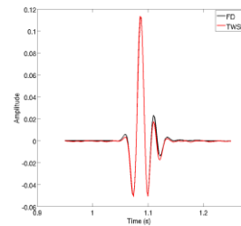
Рисунок 19. Наложение трасс МНКВ (красная) и МКР (чёрная).
