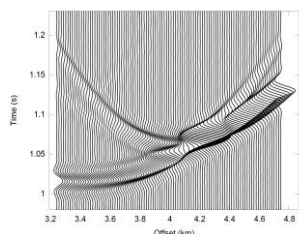
Рисунок 10. Интерференционное поле в приёмниках на «линия 1».
