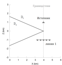
Рисунок 9. 2D сечение модели среды и система наблюдений.
