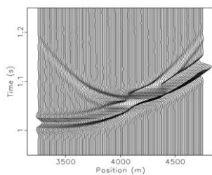
Рисунок 17. Полное волновое поле, смоделированное МКР.
