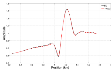
Рисунок 21. Наложение кривой КДО МНКВ на КДО МКР.
