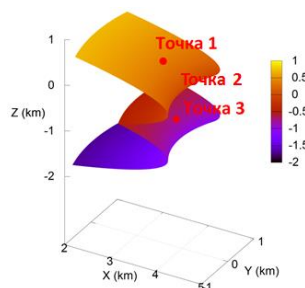
Рисунок 7. Граница типа «катушка».
