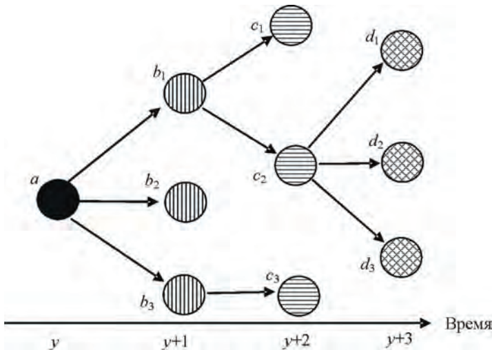
Рис. 3.6.1. Ветвление цитирования
