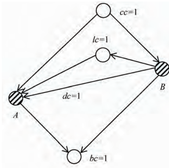
Рис. 6.4.1. Комбинированная мера
