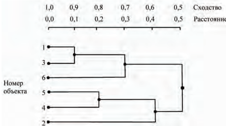
Рис. 5.5.1. Пример дендрограммы
