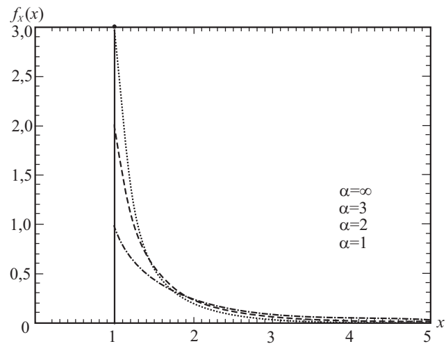
Рис. 3.2. Функция плотности вероятности (PDF)
